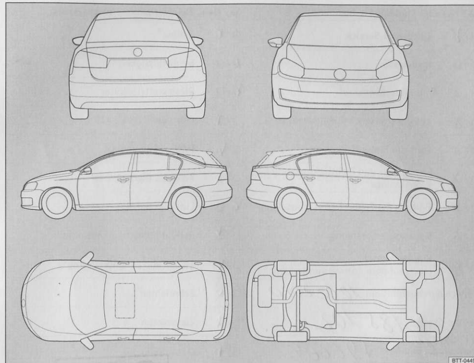
Abb. 6 Prinzipdarstellung. Gilt für alle Fahrzeuge und Karosserieformen.
